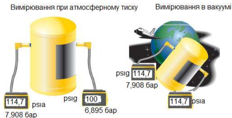
Рисунок 2.30 – Різниця при вимірі абсолютного і відносного тиску
