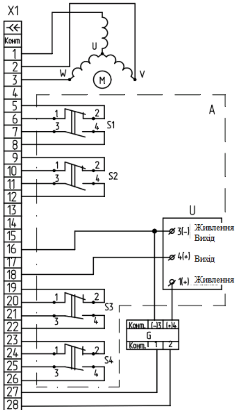
Рисунок 3.17 – Схема електрична принципова механізму МЕО-1000/63-0,63У-92КБ
