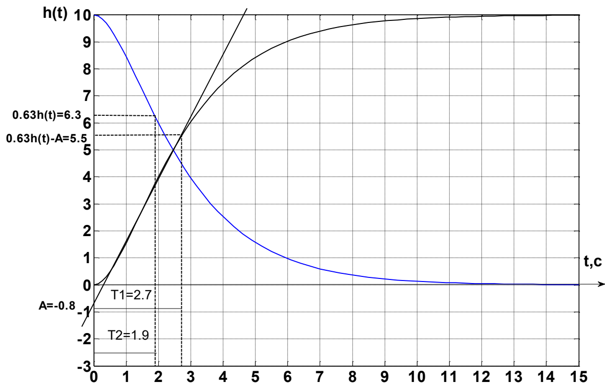
Рисунок 2.29 – Ідентифікація постійних часу за перехідною характеристикою
