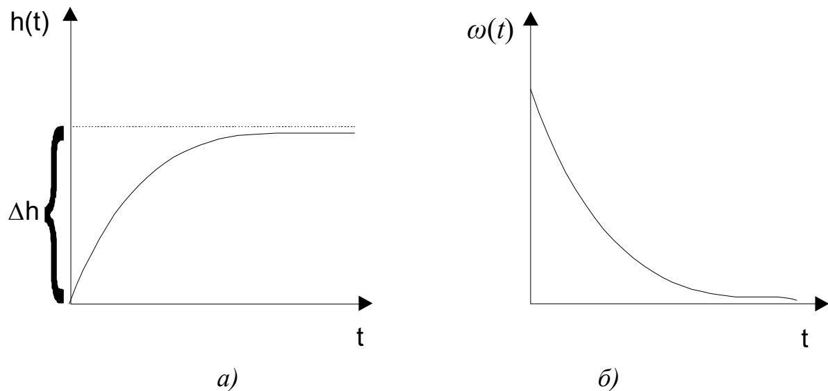
Рисунок 2.19 – Методика ідентифікації параметрів аперіодичної ланки 1-го порядку
