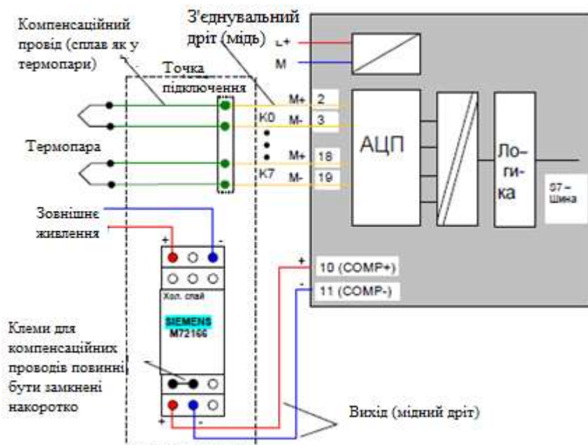
Рисунок 3.10 – Функціональна електрична схема підключення термопар з зовнішньою компенсацією температури холодного спаю до аналогового модуля SM331
