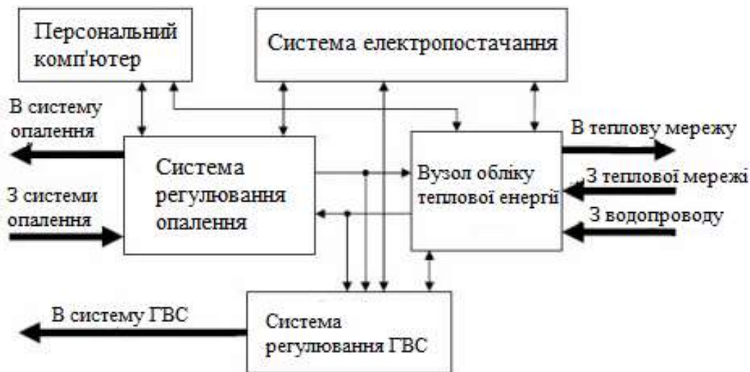
Рисунок 3.1 – Приклад оформлення структурної електричної схеми АСУ теплопостачання будівлі
