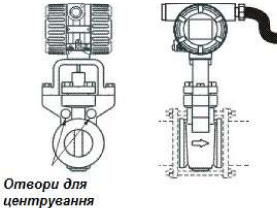
Рисунок 2.36 – Сендвічеве з'єднання датчика витрати
