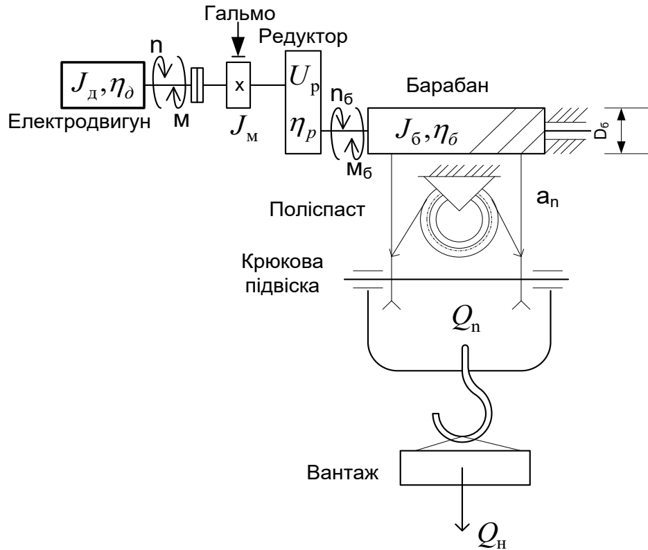
Рисунок 2.7 – Кінематична схема механізму підйому мостового крана
