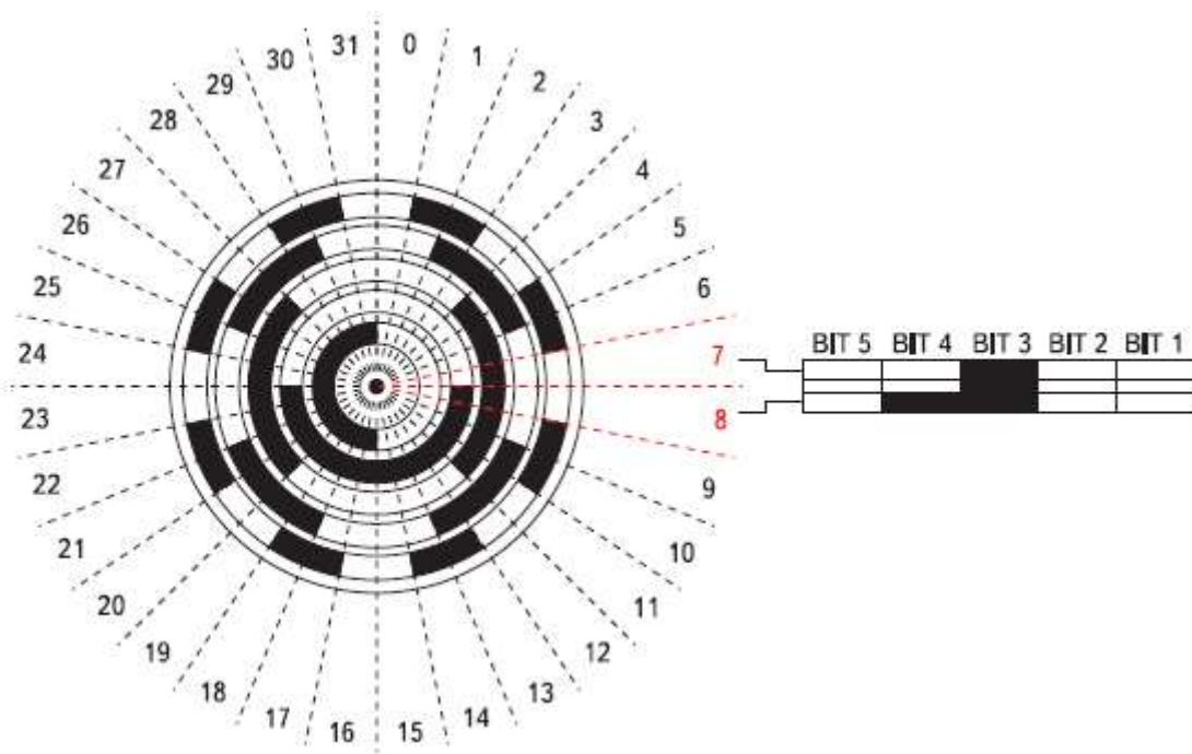
Рисунок 2.41 – Принцип створення коду положення в абсолютному датчику
