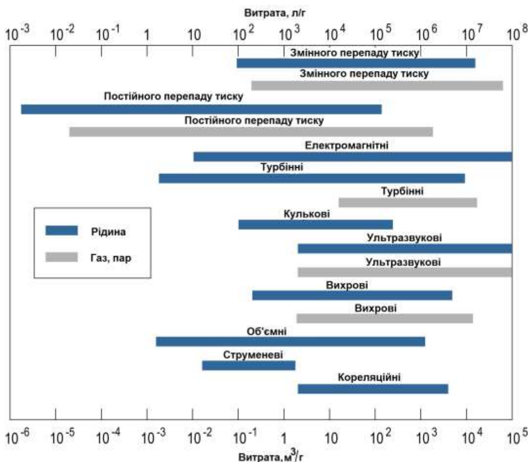
Рисунок 2.34 – Діапазони вимірювань витратомірів
