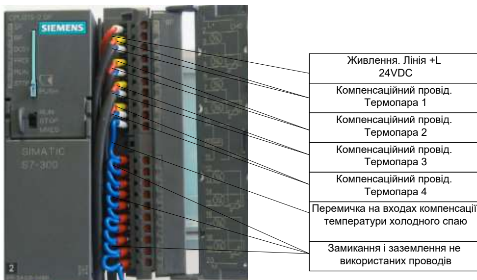
Рисунок 3.9 – Ілюстрація підключення термопар за допомогою компенсаційних проводів з внутрішньою компенсацією температури холодного спаю до модуля SM331
